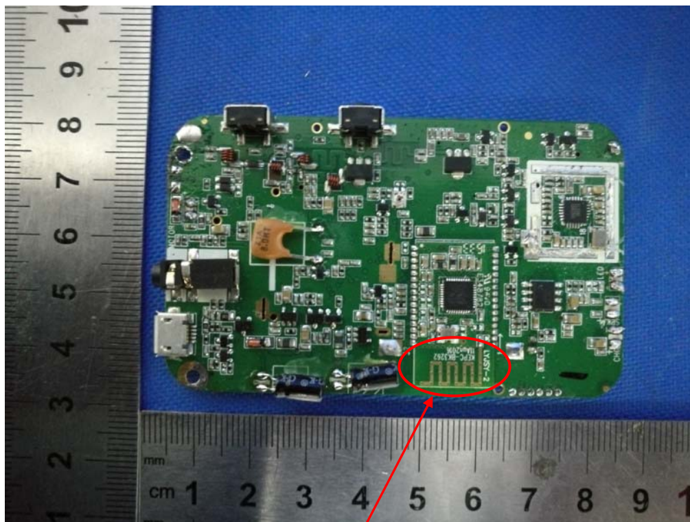
BT Ant
