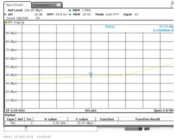
Band II 11a(HT20) CH52, AV
