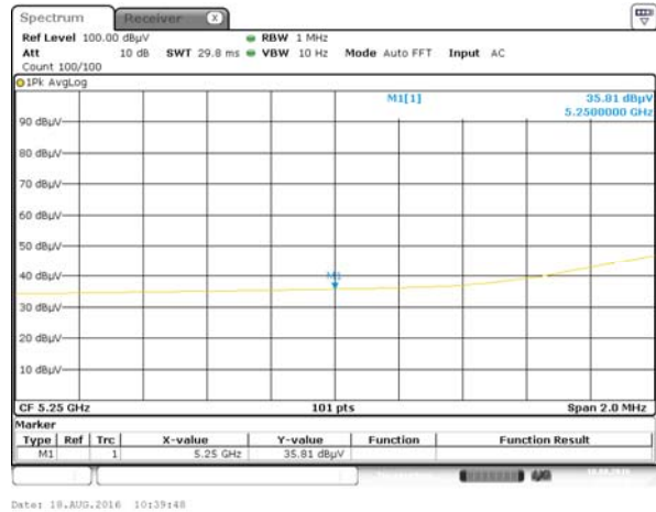
Band II 11n(HT40) CH54, AV
