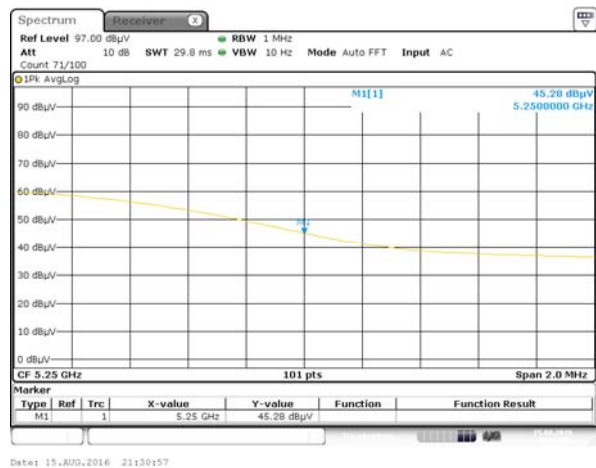
Band I 11n(HT20) CH48, AV
