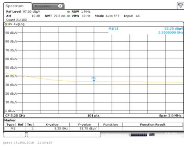
Band I 11ac(HT80) CH42, AV
