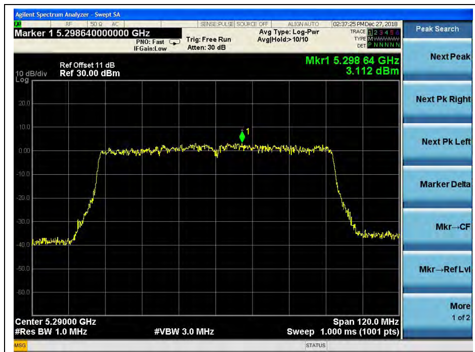
(Channel 58, 5290 MHz, 802.11 ac (VHT80), ANT0)
