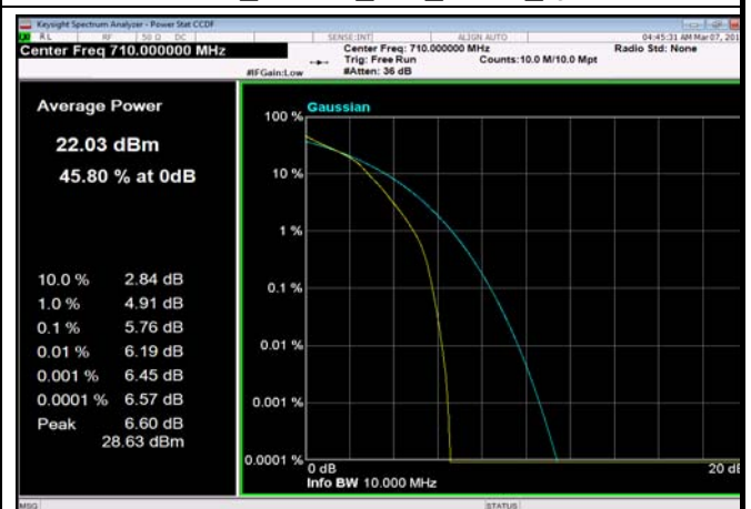
FDD17_10MHz_710_fullRB_Q16
