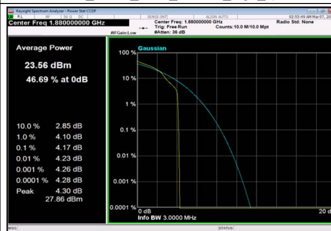
FDD02_5MHz_1880_OneRB_high_Q16
