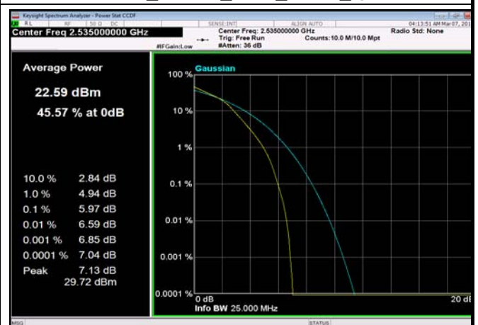
FDD07_20MHz_2535_fullRB_Q16
