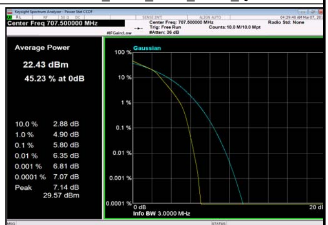
FDD12_3MHz_707.5_fullRB_Q16
