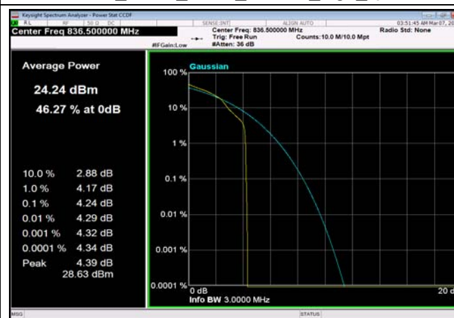
FDD05_5MHz_836.5_OneRB_high_Q16
