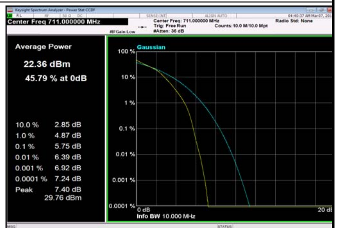
FDD12_10MHz_711_fullRB_Q16
