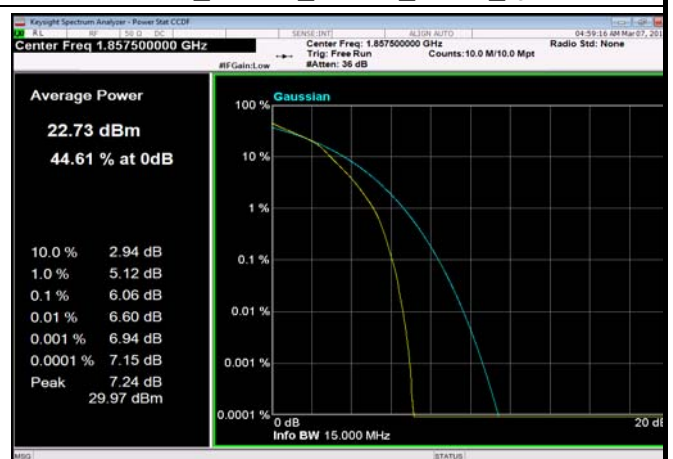
FDD25_15MHz_1857.5_fullRB_Q16
