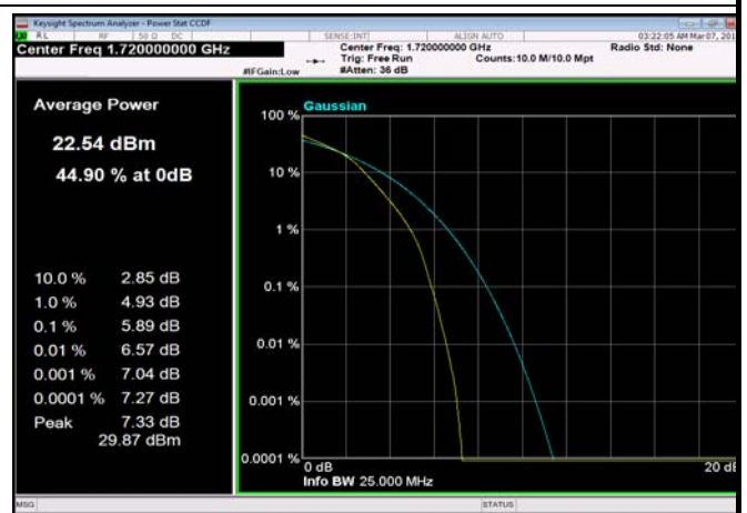
FDD04_20MHz_1720_fullRB_Q16
