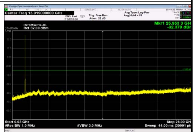
FDD25_HighRange_5MHz_30MHz~26GHz
