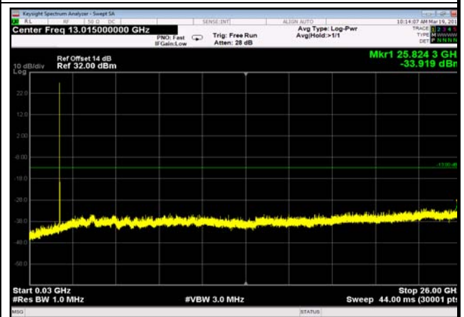
FDD25_LowRange_20MHz_30MHz~26GHz
