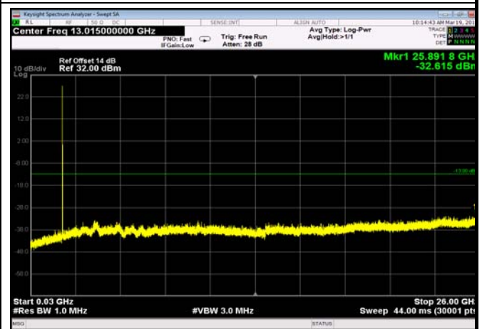
FDD25_MidRange_20MHz_30MHz~26GHz
