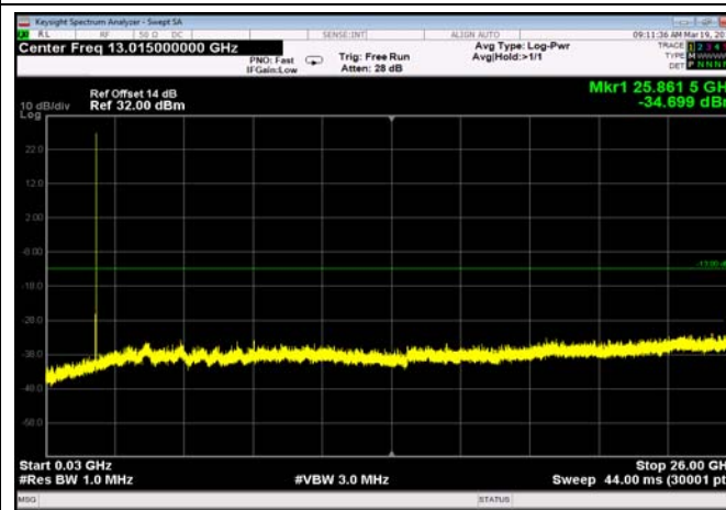
FDD25_HighRange_15MHz_30MHz~26GHz
