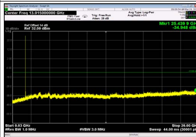
FDD25_LowRange_15MHz_30MHz~26GHz
