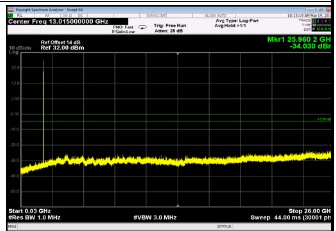
FDD25_HighRange_20MHz_30MHz~26GHz
