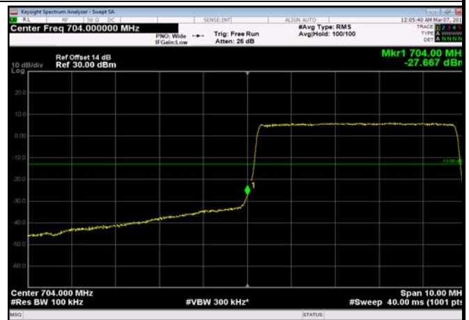
LowRange_FDD17_10MHz_709_OneRB _low_Q16
