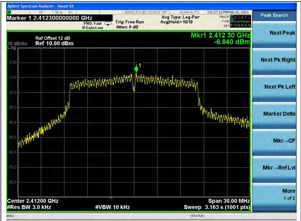
(Channel 1, 802.11g, ANT0)
