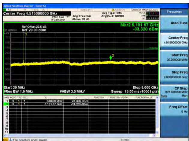
Band19 / 10MHz / Low CH / 16QAM
