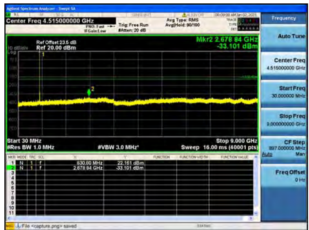
Band19 / 10MHz / Low CH / 64QAM
