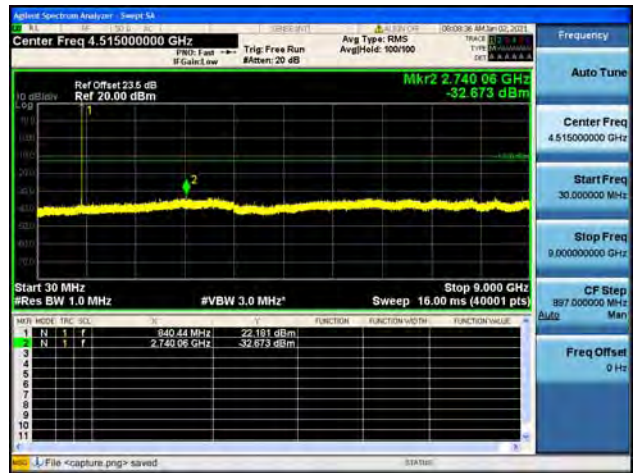
Band19 / 10MHz / Low CH / QPSK
