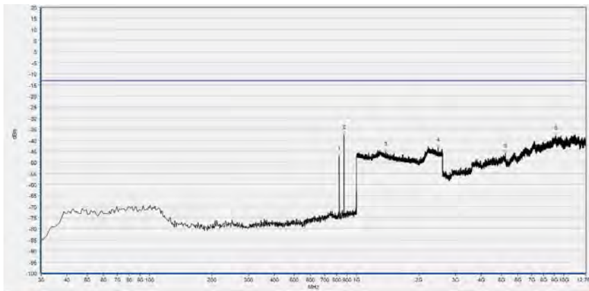
CDMA2000 BC0 (1xRTT), Low Channel
