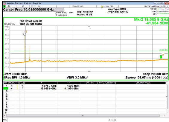
B2_n41(90M)_DFT-s-OFDM_BPSK_Edge_ 1RB_Left_Low_CH
