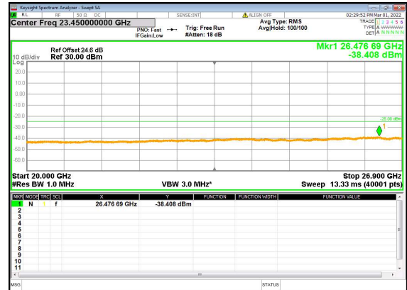
B2_n41(90M)_DFT-s-OFDM_BPSK_Edge_ 1RB_Left_Low_CH
