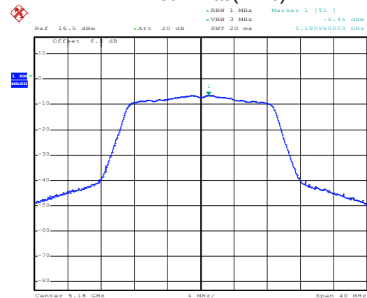
802.11ac(HT20)
