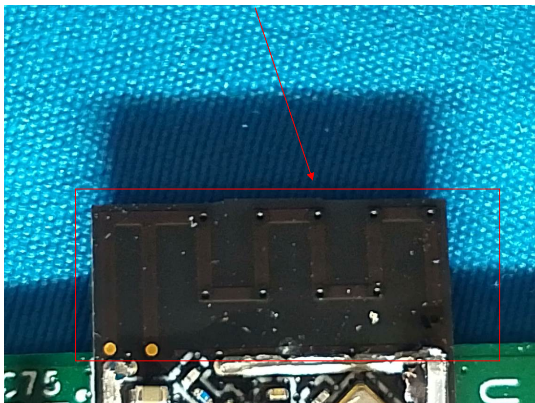
BLE/WIFI Antenna
