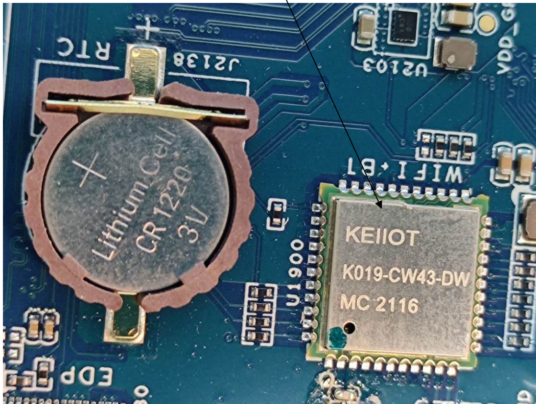
WiFi&Bluetooth Module
