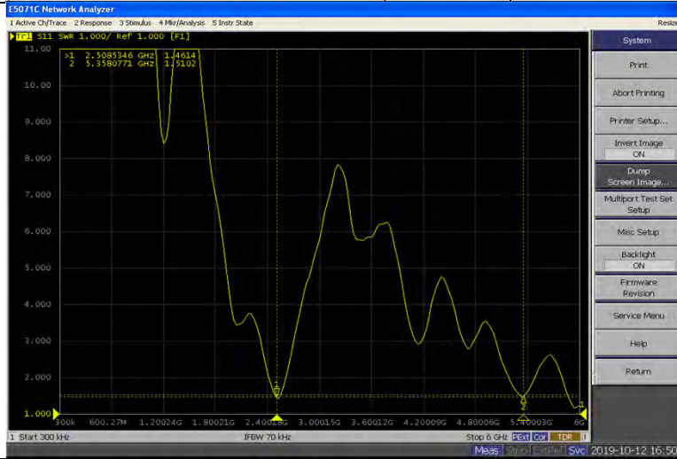
VSWR
