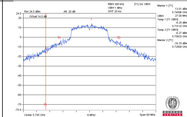
802.11a_Chain3 / CH149
