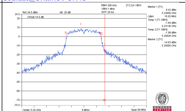
802.11ac(VHT20)_Chain1 / CH48
