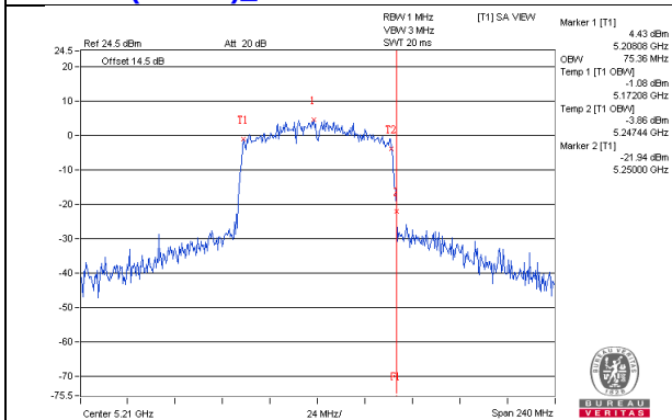
802.11ac(VHT80)_Chain2 / CH42
