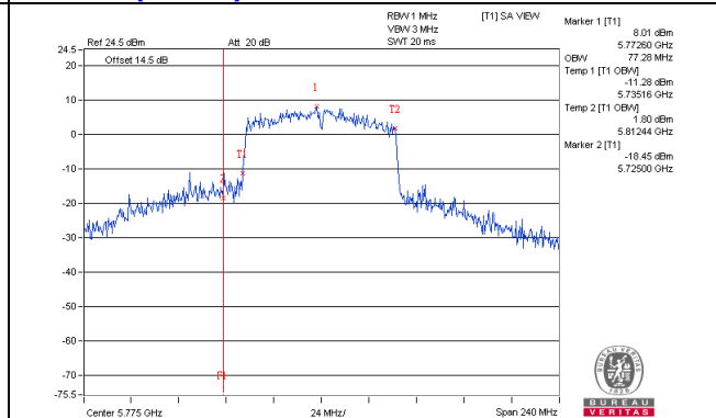
802.11ac(VHT80)_Chain3 / CH155
