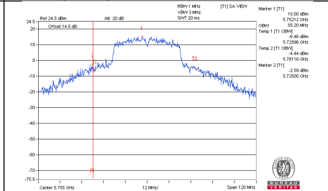
802.11ac(VHT40)_Chain3 / CH151
