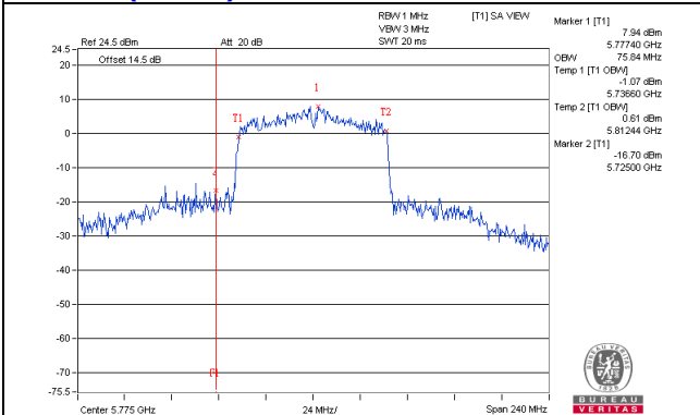
802.11ac(VHT80)_Chain2 / CH155
