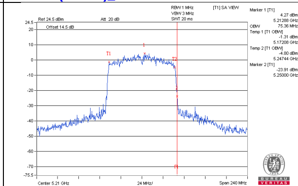
802.11ac(VHT80)_Chain3 / CH42
