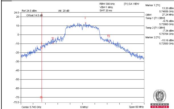
802.11a_Chain2 / CH149
