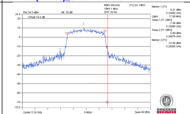
802.11ac(VHT20)_Chain3 / CH48
