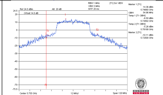
802.11ac(VHT80)_Chain1 / CH155
