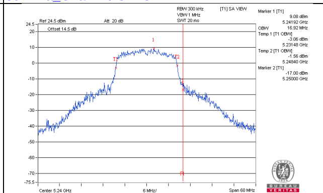
802.11a_Chain3 / CH48
