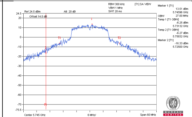
802.11a_Chain3 / CH149
