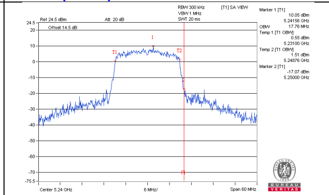
802.11ac(VHT20)_Chain3 / CH48
