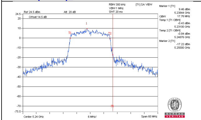
802.11ac(VHT20)_Chain2 / CH48
