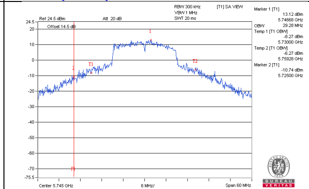
802.11ac(VHT20)_Chain3 / CH149
