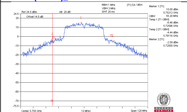
802.11ac(VHT40)_Chain3 / CH151
