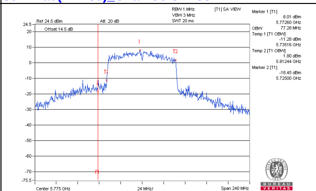
802.11ac(VHT80)_Chain3 / CH155
