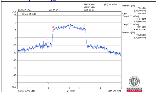
802.11ac(VHT80)_Chain2 / CH155
