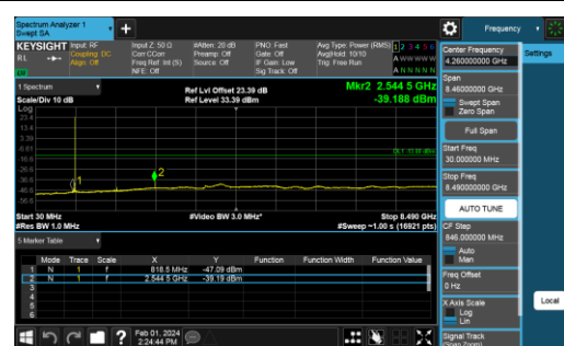
B5-10M-Low CH-CSE-1-Q16-1 RB 0
