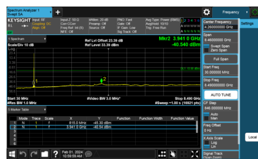
B5-3M-Mid CH-CSE-1-Q16-1 RB 0
