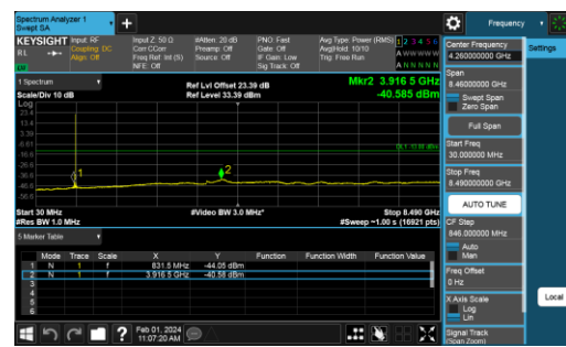
B5-3M-Low CH-CSE-1-Q16-1 RB 0
