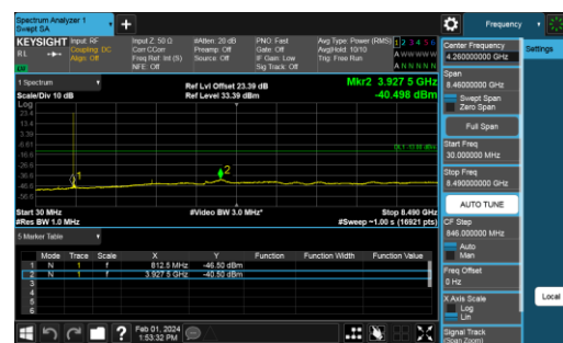
B5-5M-Mid CH-CSE-1-Q16-1 RB 0
