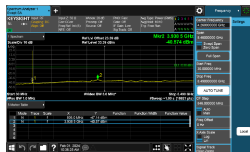
B5-1.4M-Mid CH-CSE-1-Q16-1 RB 0
