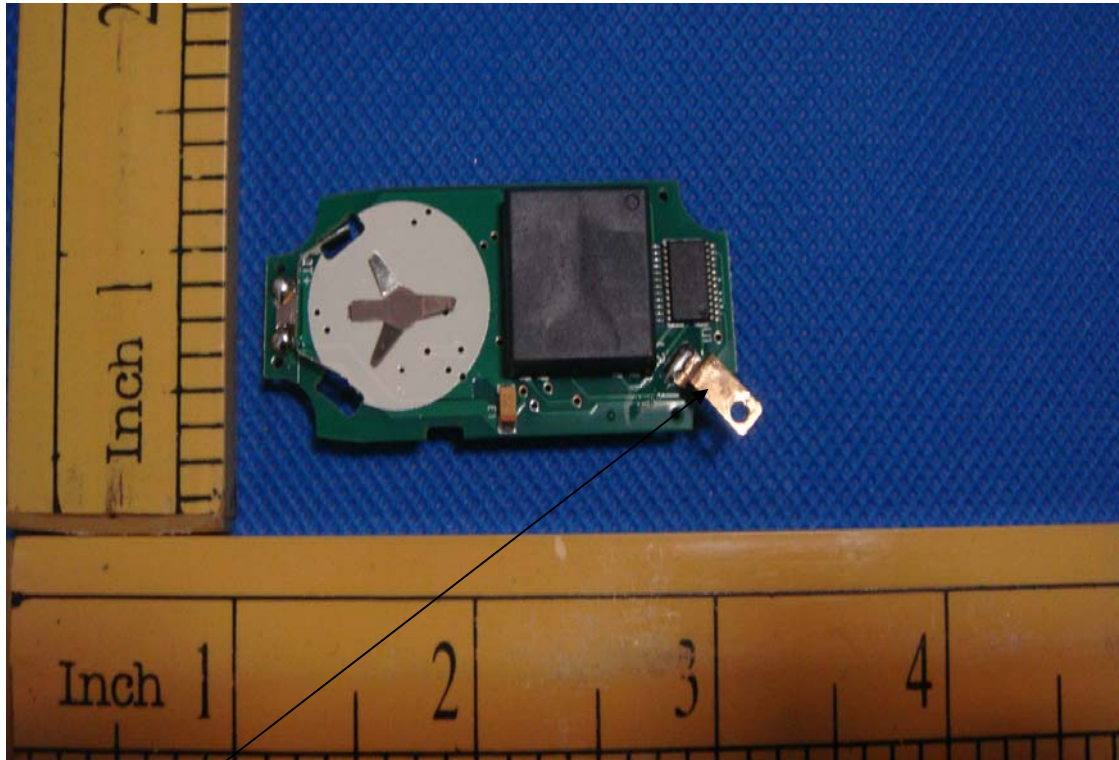
Antenna
