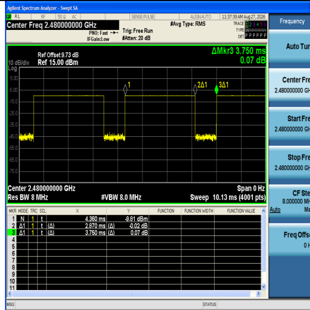
NTNV-DH5-Ant1-2480
