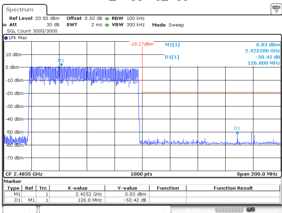
DH1_Hopping_Upper
