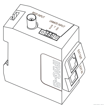
Figure 126 - IRIG-B module
