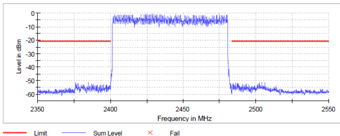
Band Edge
