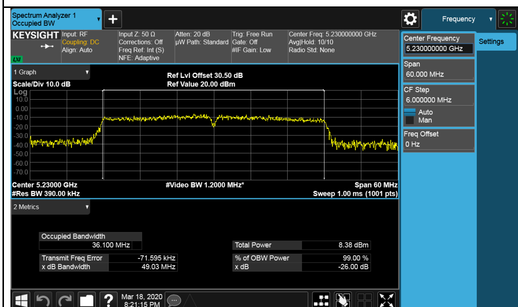
802.11n-HT40-5230MHz
