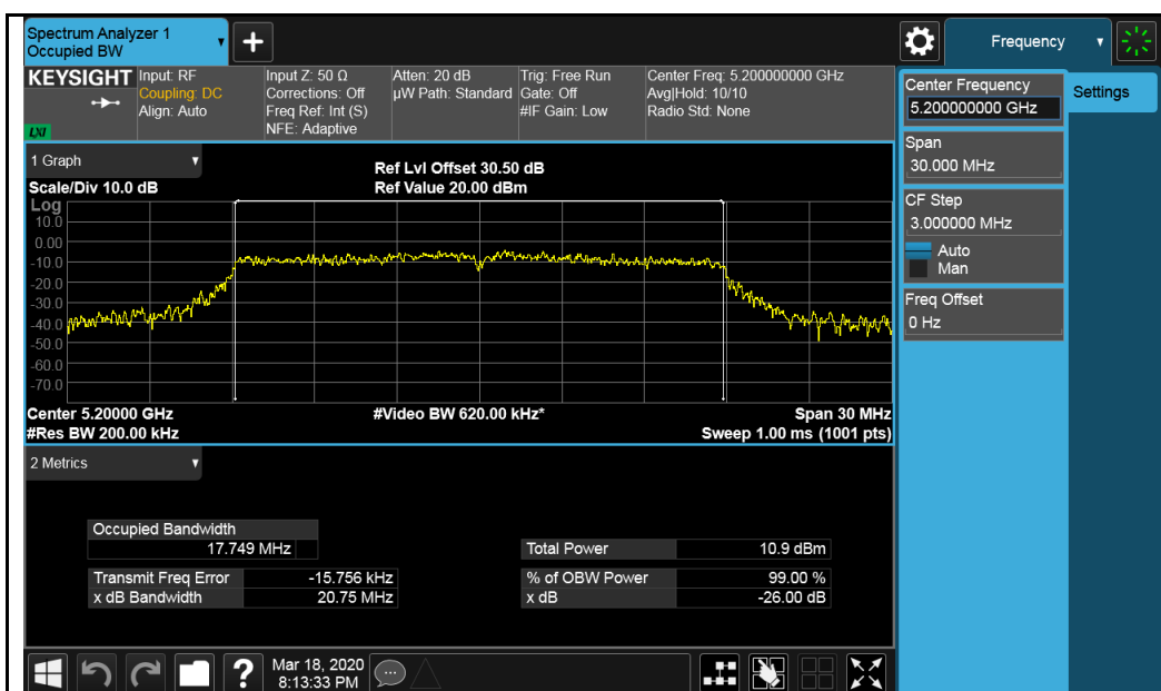
802.11n-HT20-5200MHz
