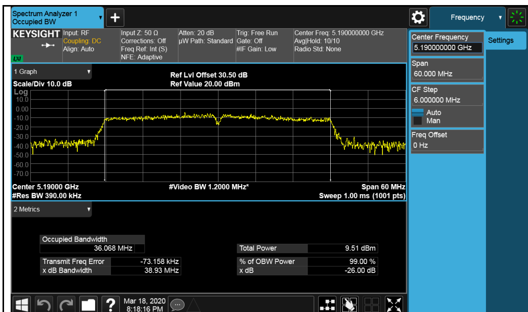
802.11n-HT40-5190MHz
