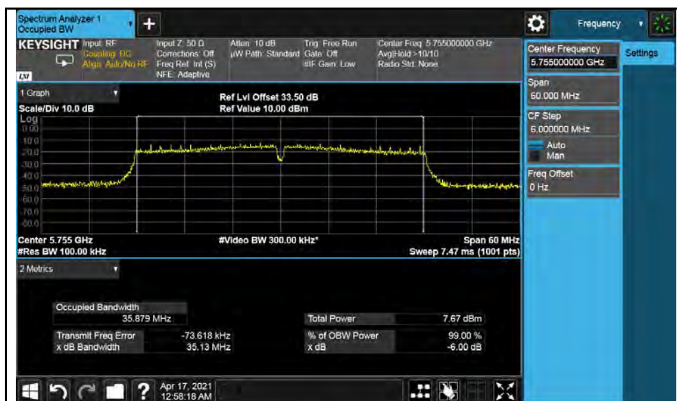
802.11n-HT40-5755MHz
