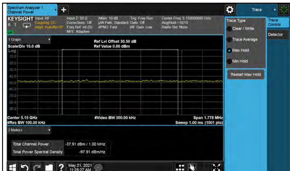
802.11ac(VHT40)-5190MHz
