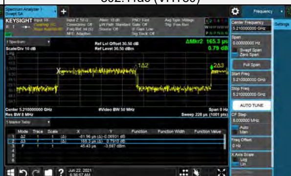
802.11ac (VHT80)
