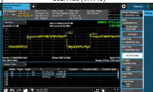
802.11ac (VHT40)
