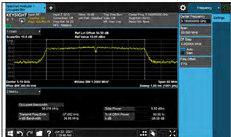
802.11n-HT40-5190MHz
