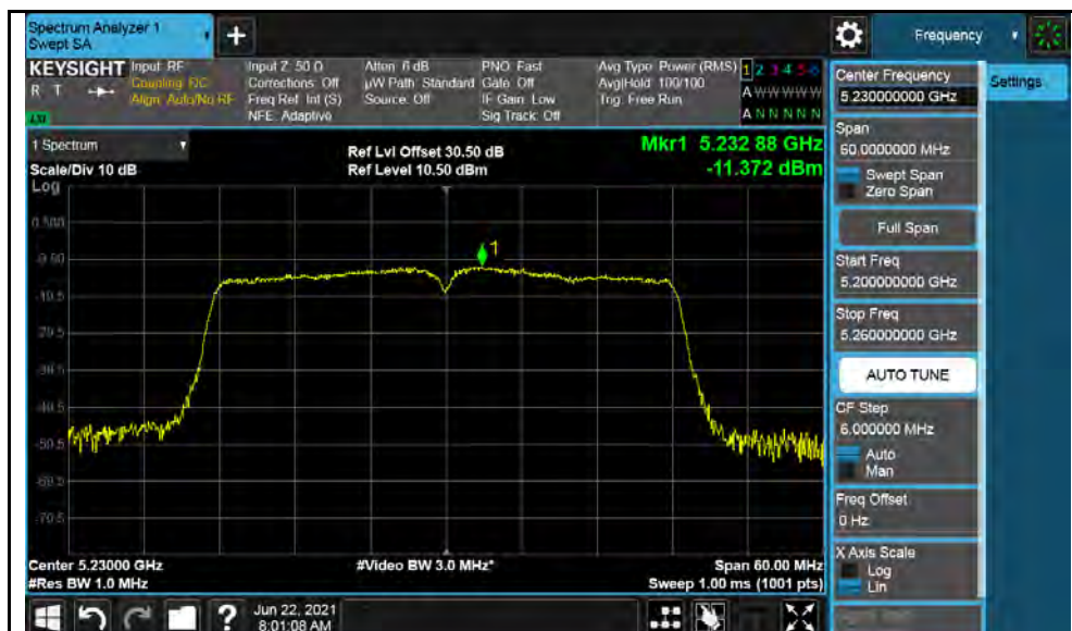
802.11n-HT40-5230MHz
