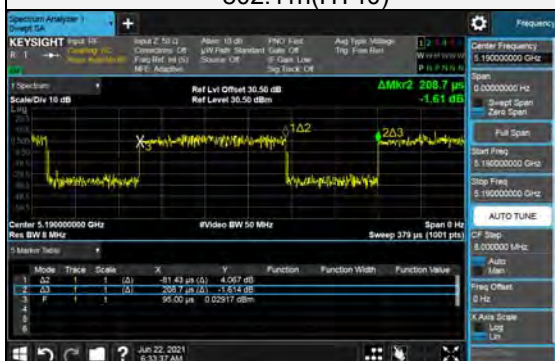
802.11n(HT40)
