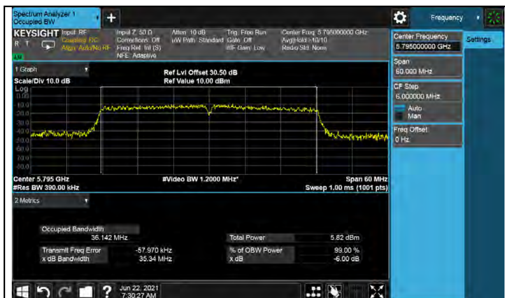
802.11n-HT40-5795MHz
