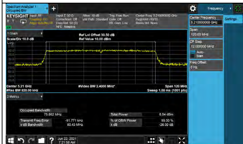
802.11ac-VHT80-5210MHz
