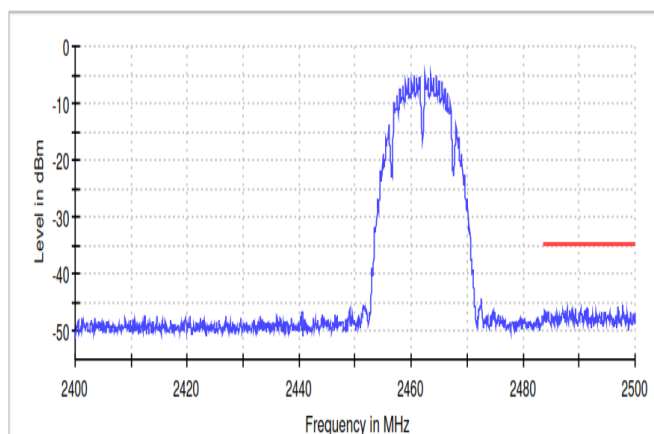
Band Edge
