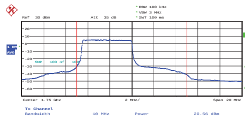
10 MHz – Ch: 20350– RB# 25 RB Pos: 0
