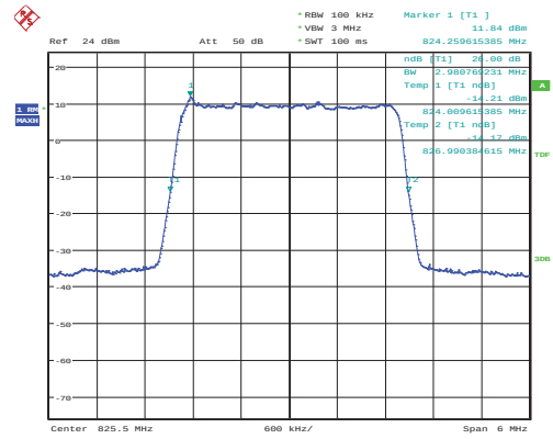
3 MHz – Ch: 20415 – QPSK
