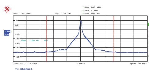
10 MHz – Ch: 20350– RB# 1 RB Pos: 25
