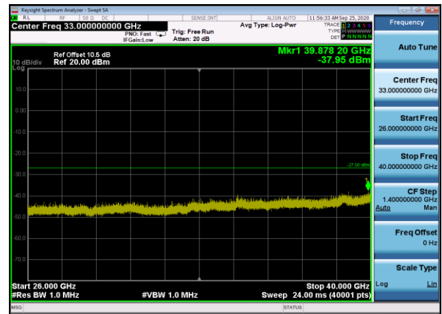
U-NII-1 ,Plot 2,26000MHz~40000MHz-802.11n(20MHz),5240MHz,Ant1
