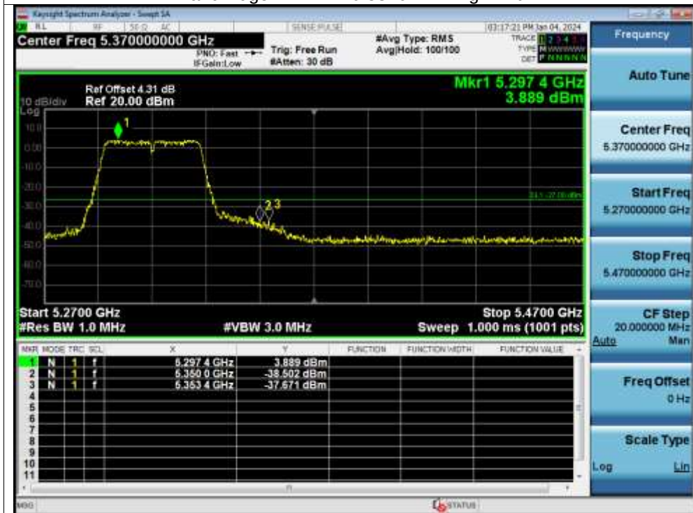
Band Edge NVNT n40 5310MHz High Ant1
