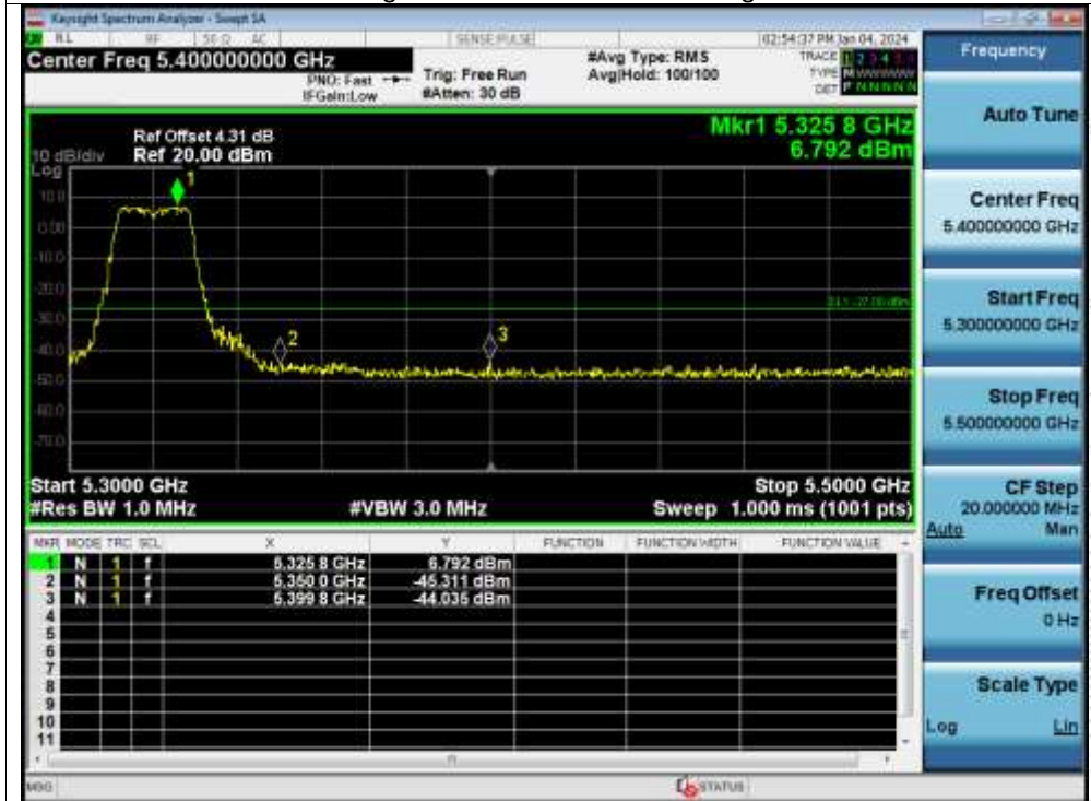
Band Edge NVNT ac20 5320MHz High Ant1
