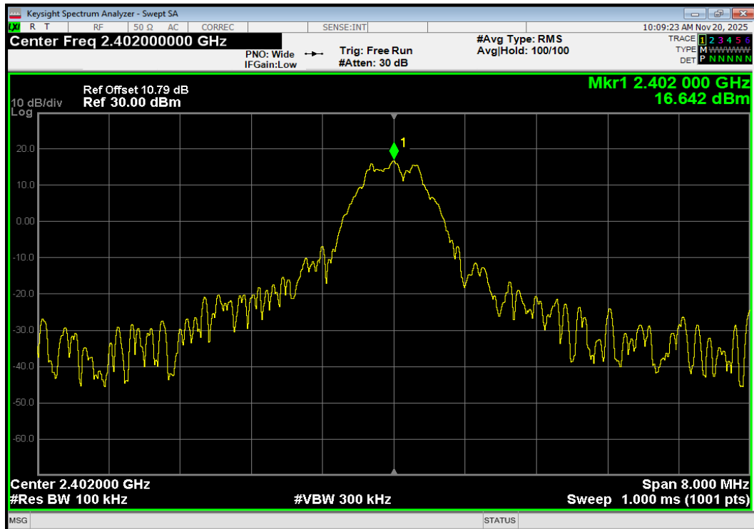
Band Edge BLE (1M)2402MHz Emission
