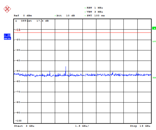
LTE Band 4 5MHz CH-Middle 3GHz~18GHz
