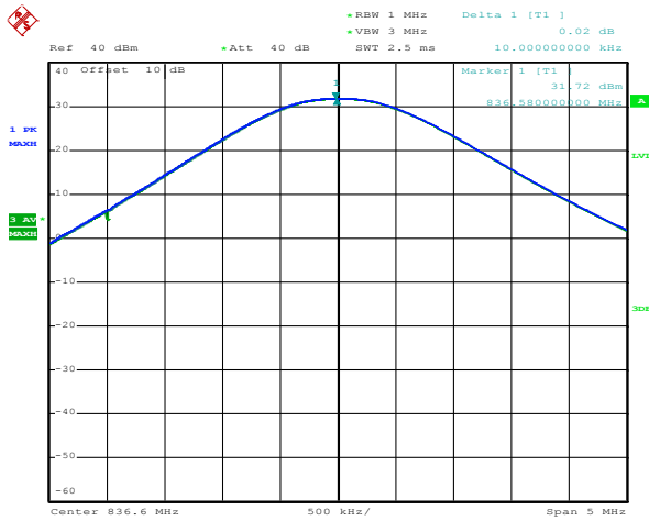
GSM 850
