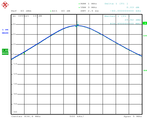
EGPRS 850
