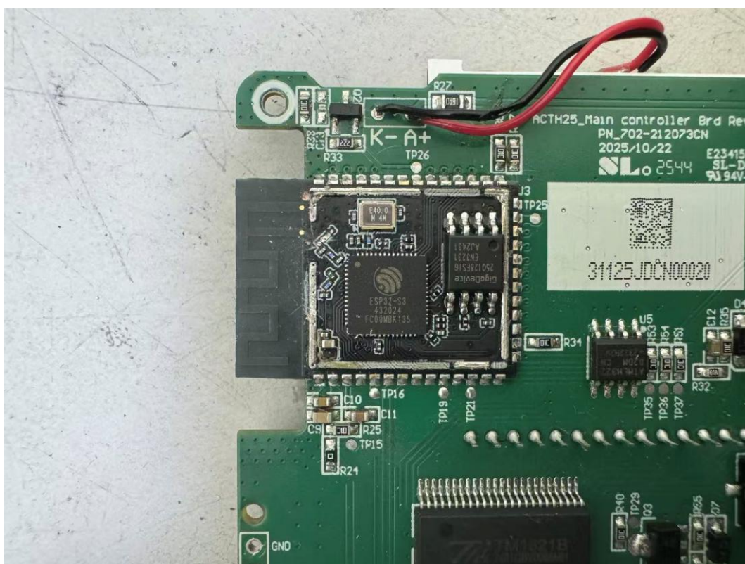
RF Module
