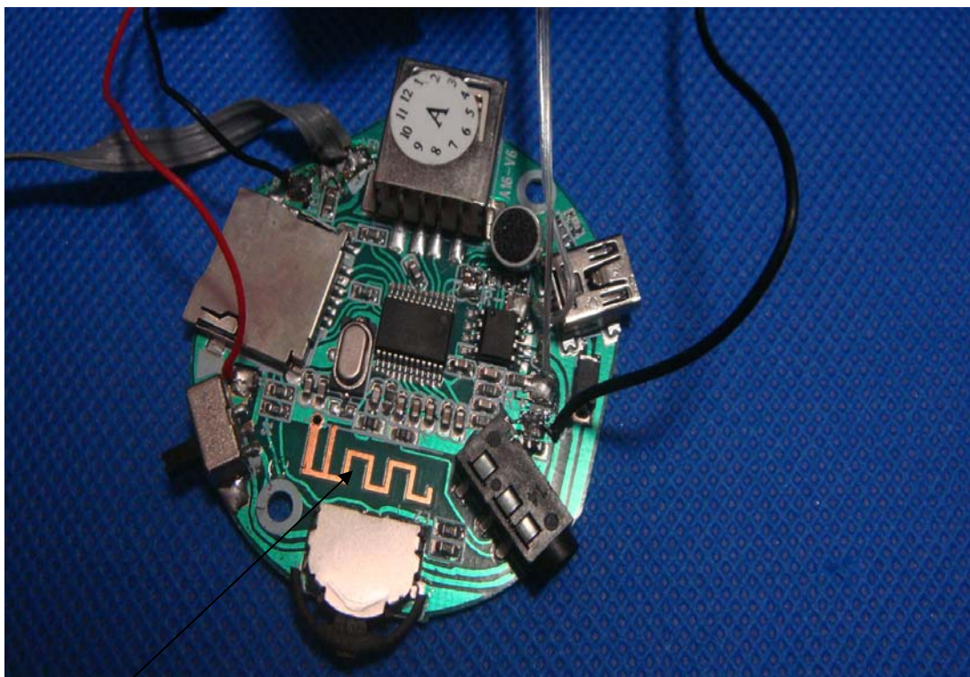
Antenna
