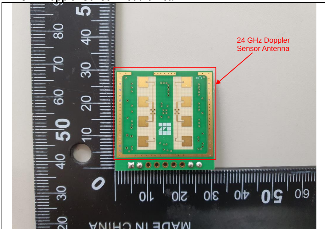
24 GHz Doppler Sensor Module Rear
