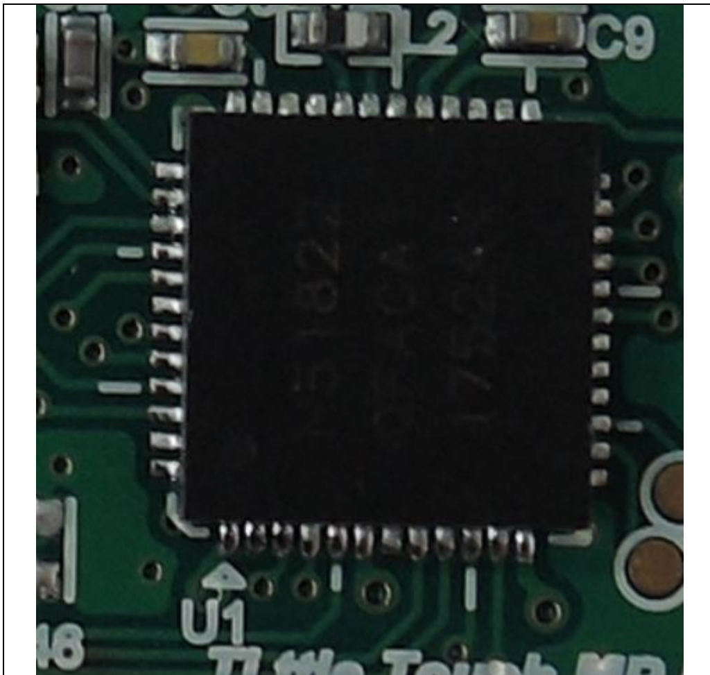
&lt;Module&gt;
