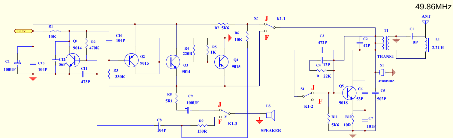
对讲机原理图-49M
