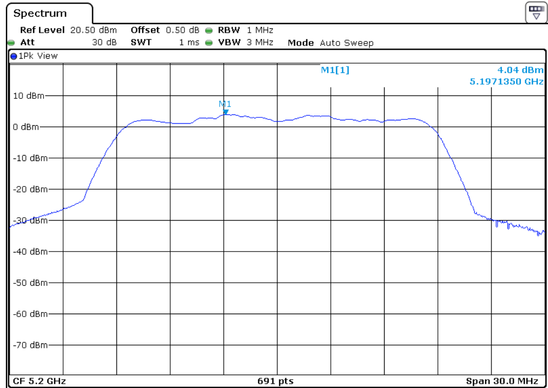
5200MHz-Ant4
