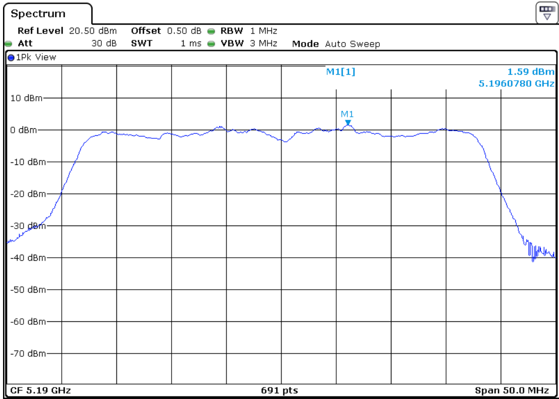
5190MHz-Ant4
