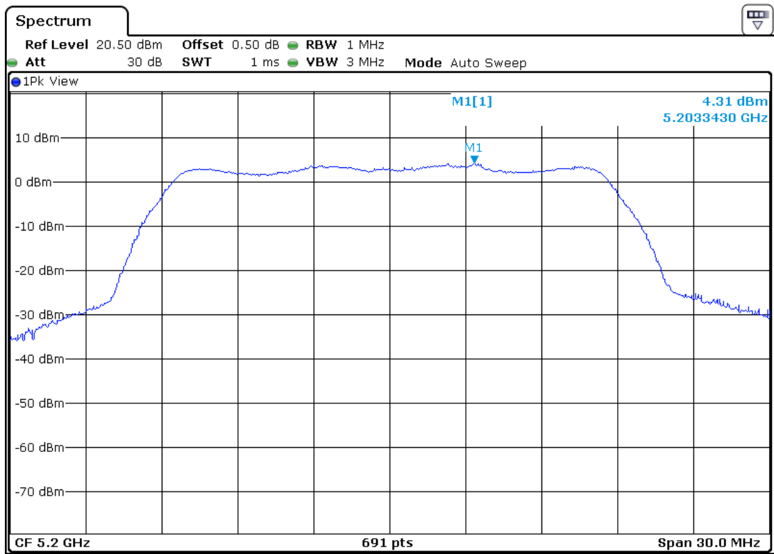
5200MHz-Ant2
