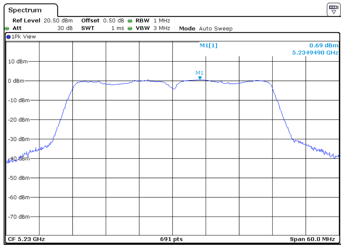
5230MHz-Ant2
