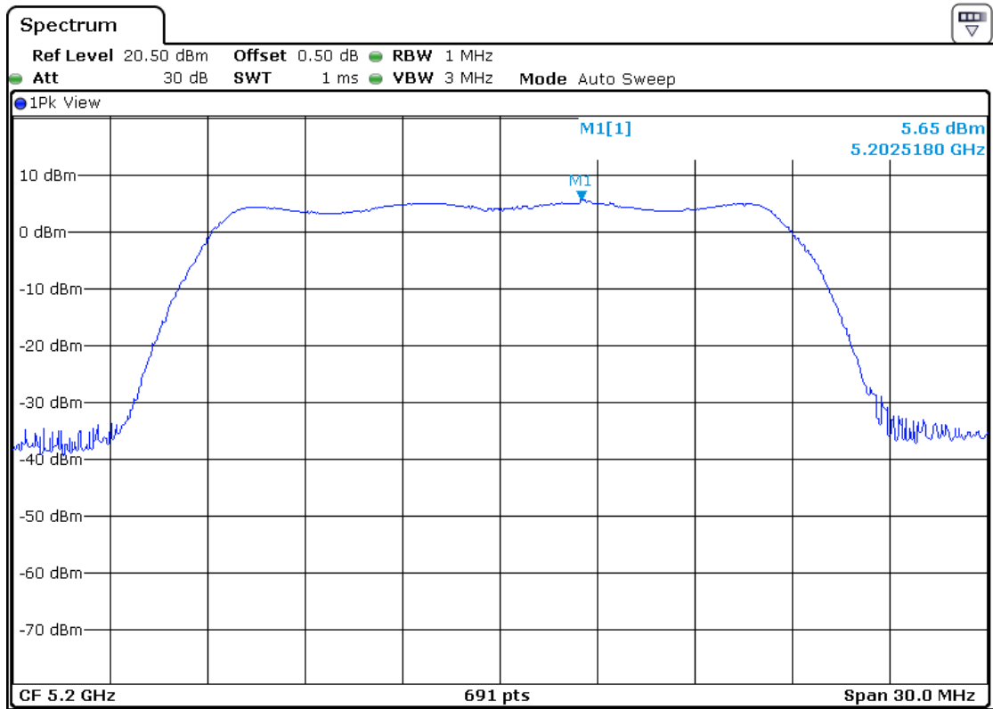
5200MHz-Ant2
