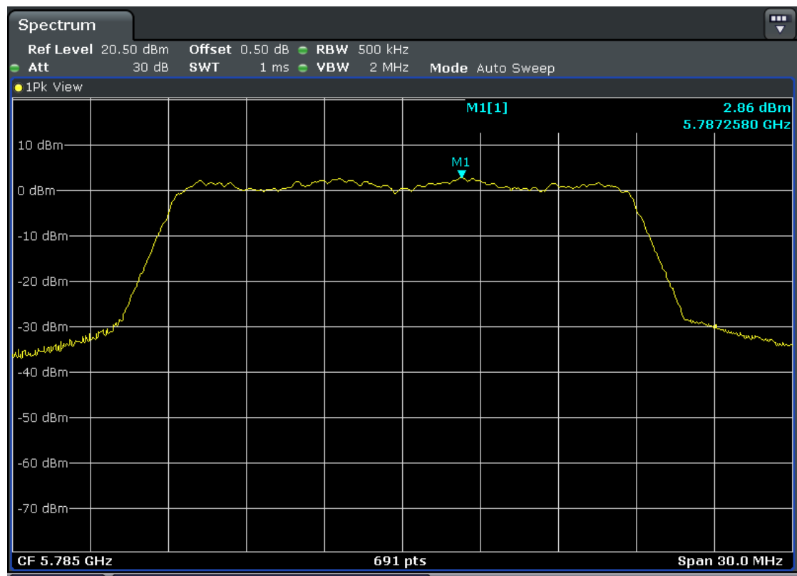
5785MHz – Ant2
