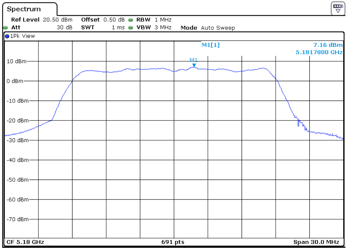
5180MHz-Ant1
