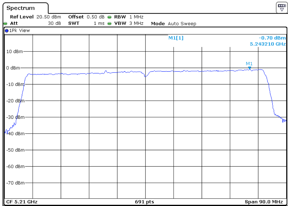
5210MHz-Ant2
