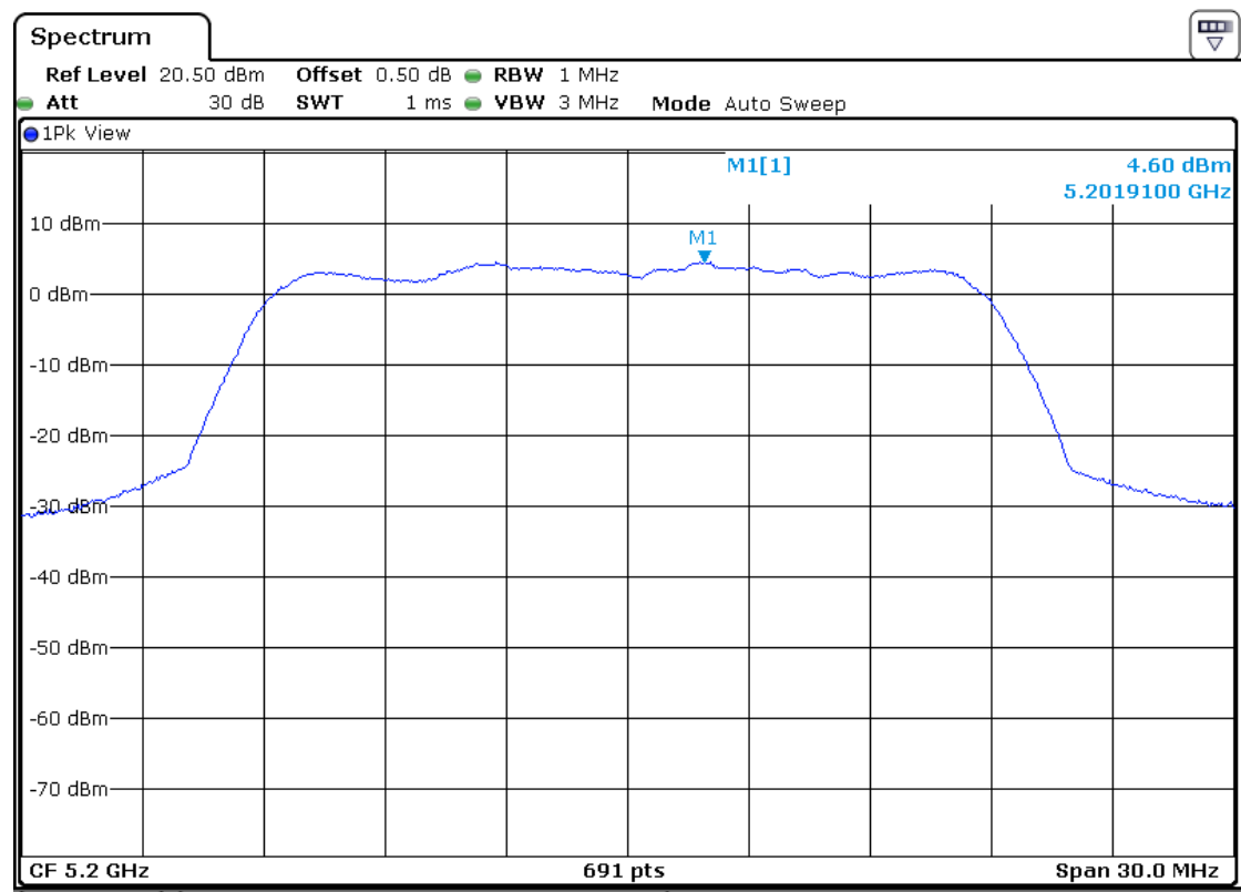
5200MHz-Ant4
