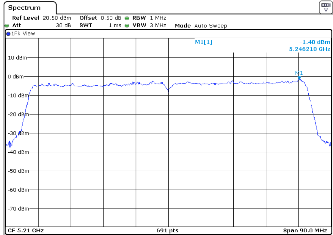
5210MHz-Ant4
