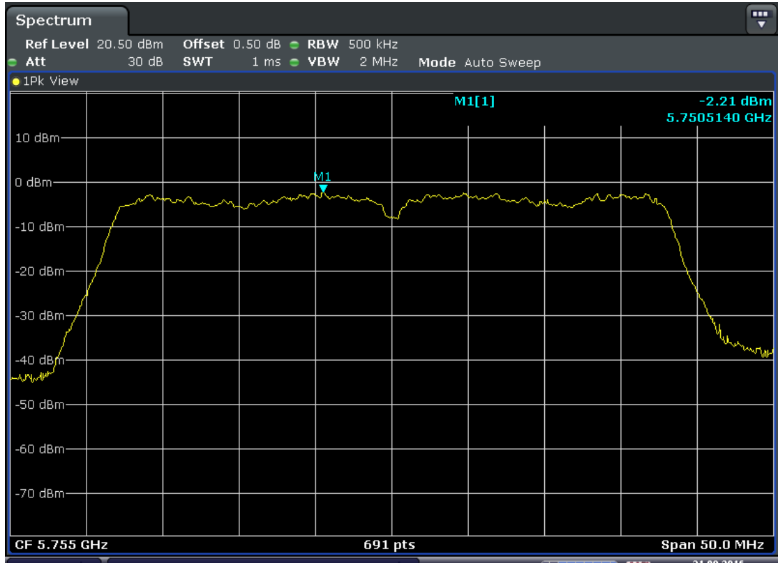
5755MHz-Ant2
