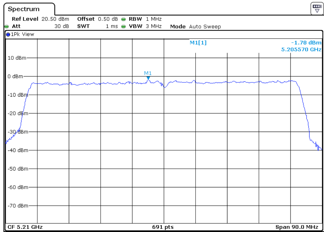
5210MHz-Ant4
