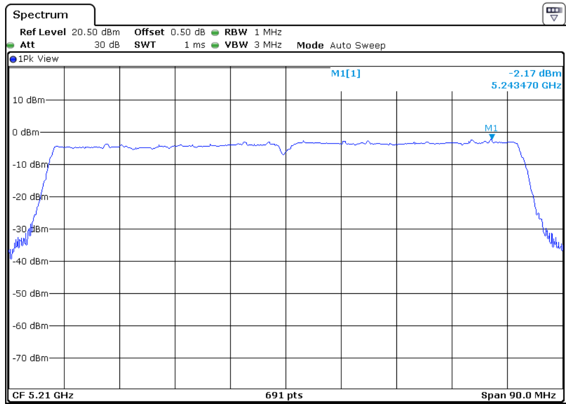
5210MHz-Ant1
