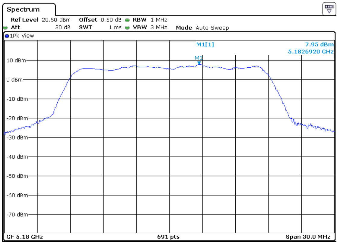
5180MHz-Ant2
