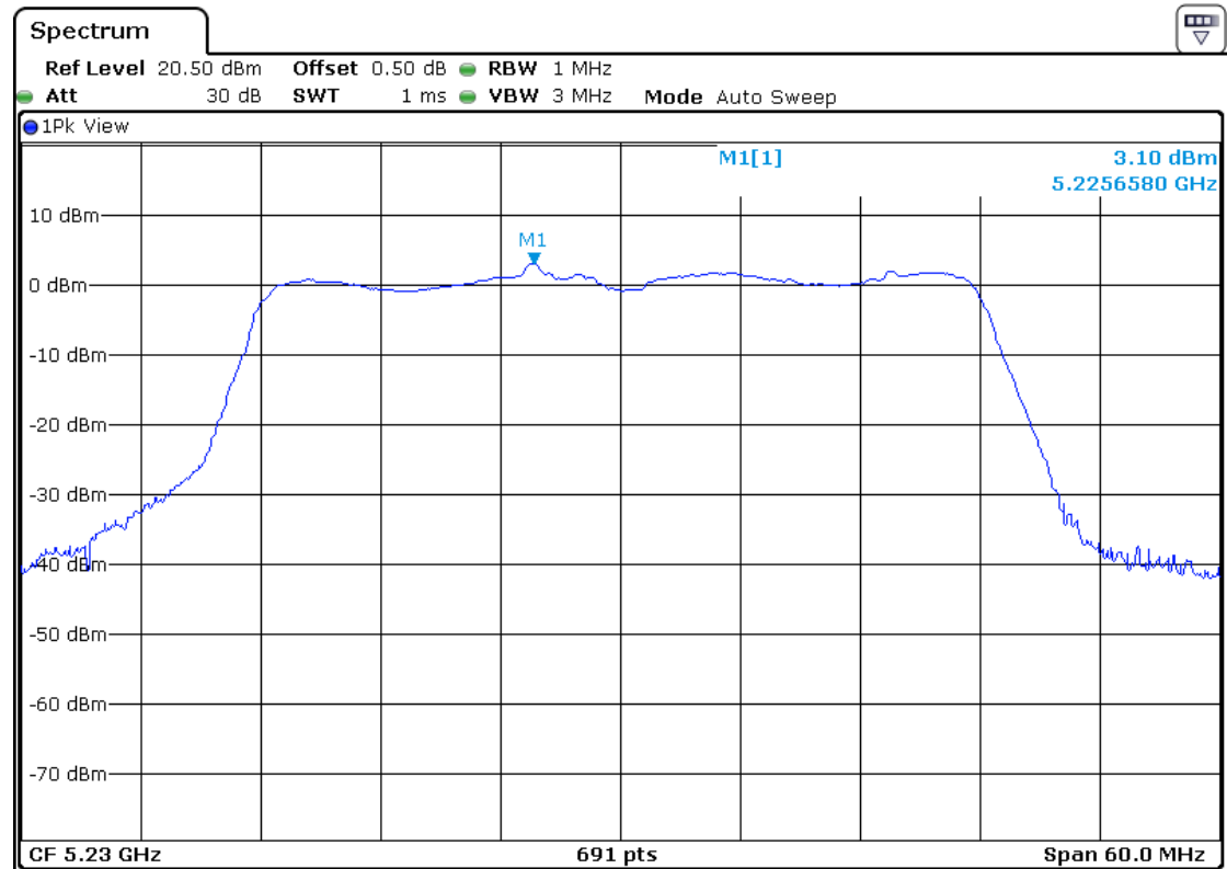
5230MHz-Ant2
