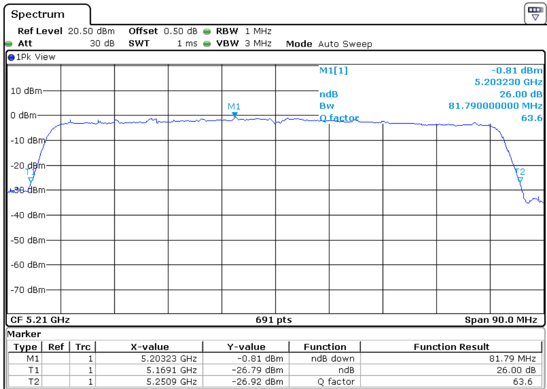
5210MHz-Ant4
