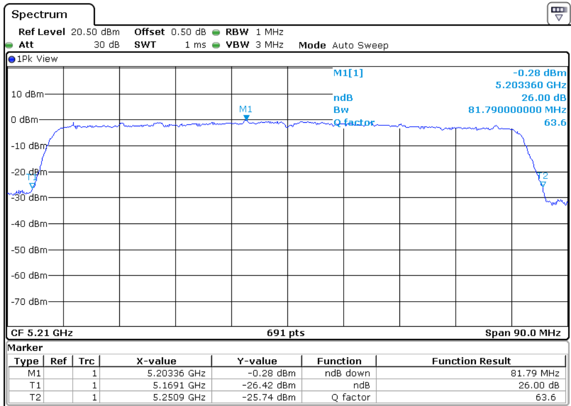
5210MHz-Ant4
