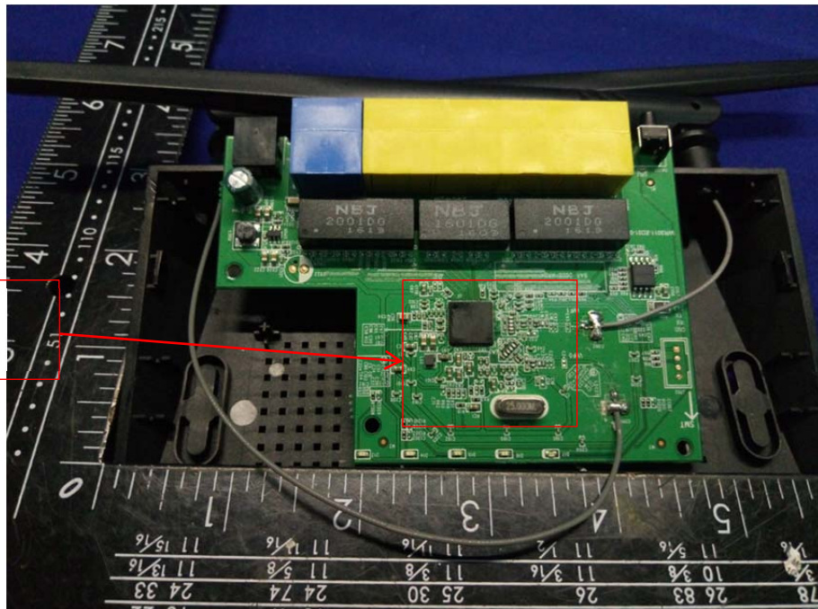
WiFi Module
