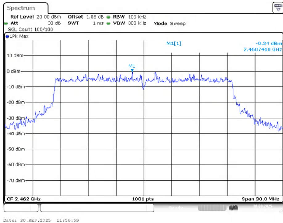
Band Edge NVNT ax20 2462MHz Ant1 Ref
