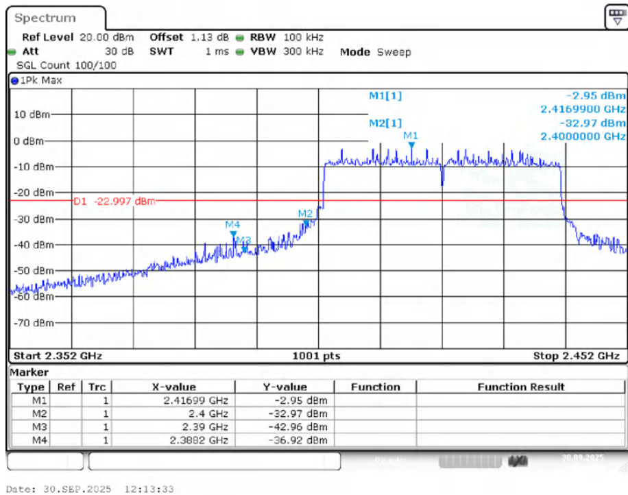
Band Edge NVNT ax40 2422MHz Ant1 Emission
