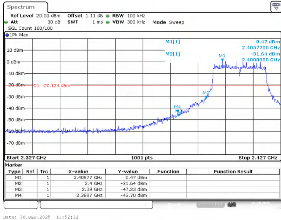
Band Edge NVNT ax20 2412MHz Ant1 Emission
