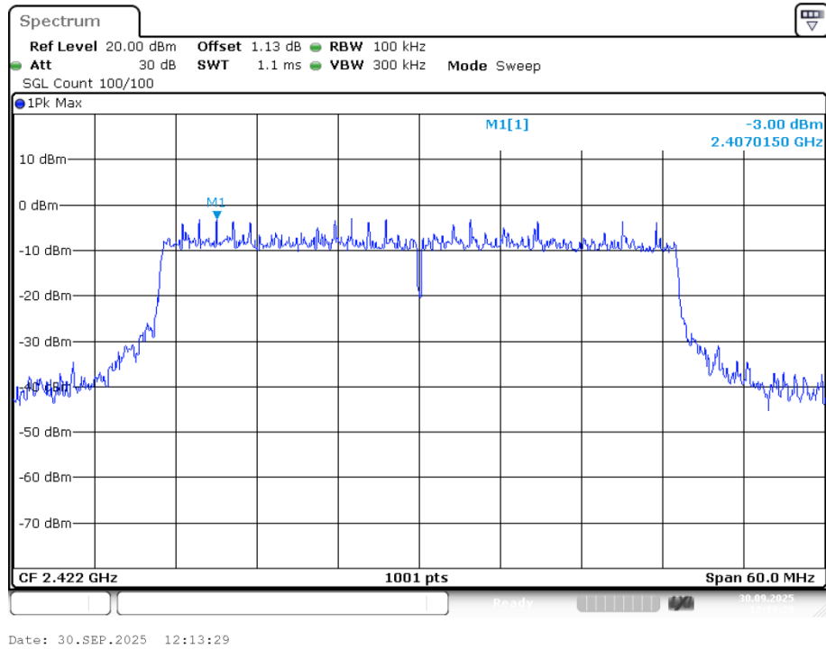
Band Edge NVNT ax40 2422MHz Ant1 Ref
