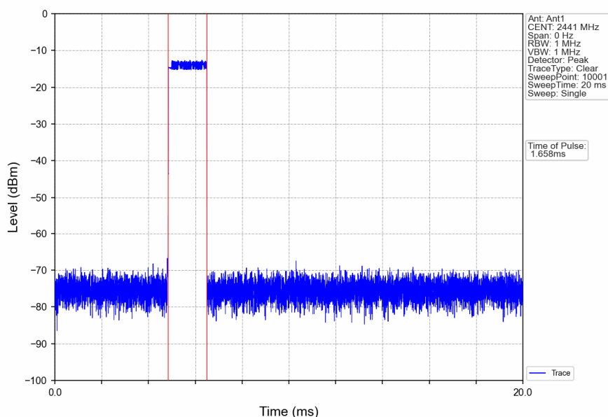
Pi/4DQPSK_2DH3_HOPP_Ant1_NTNV
