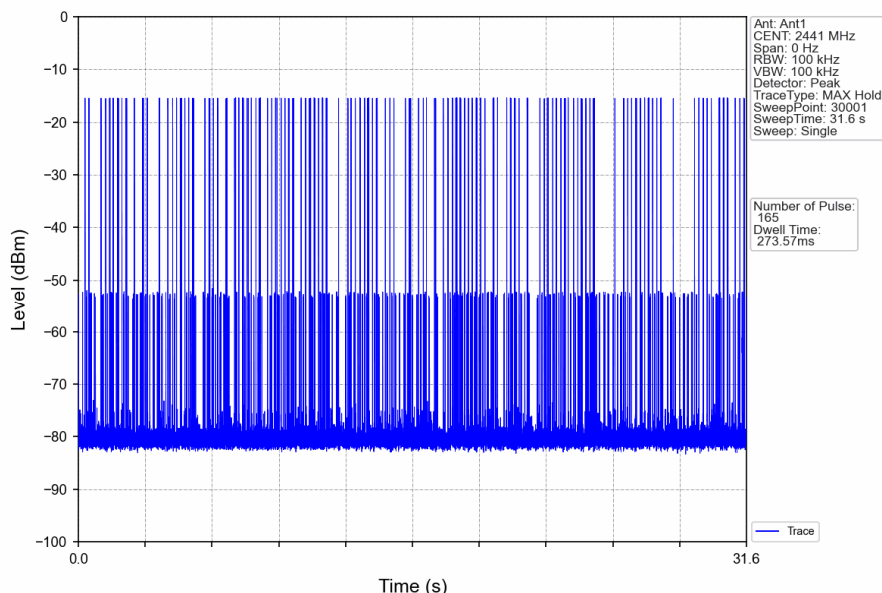
Pi/4DQPSK_2DH3_HOPP_Ant1_NTNV
