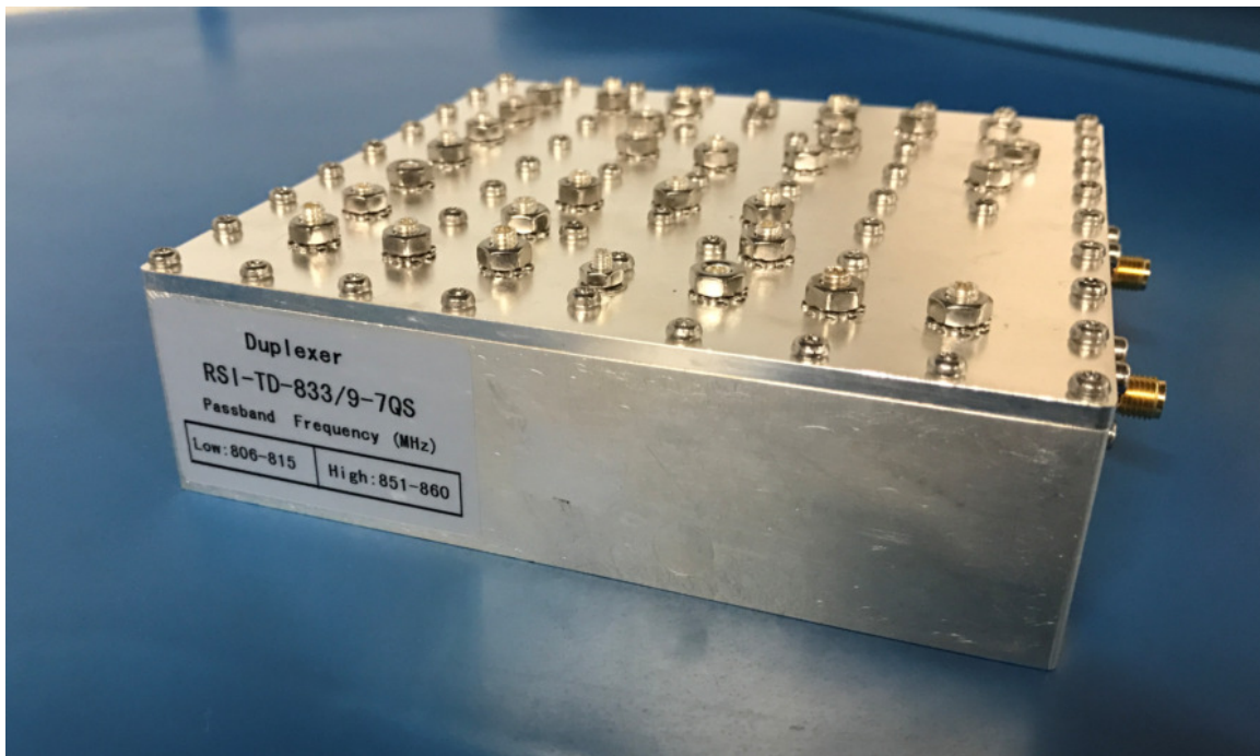
Duplexer
