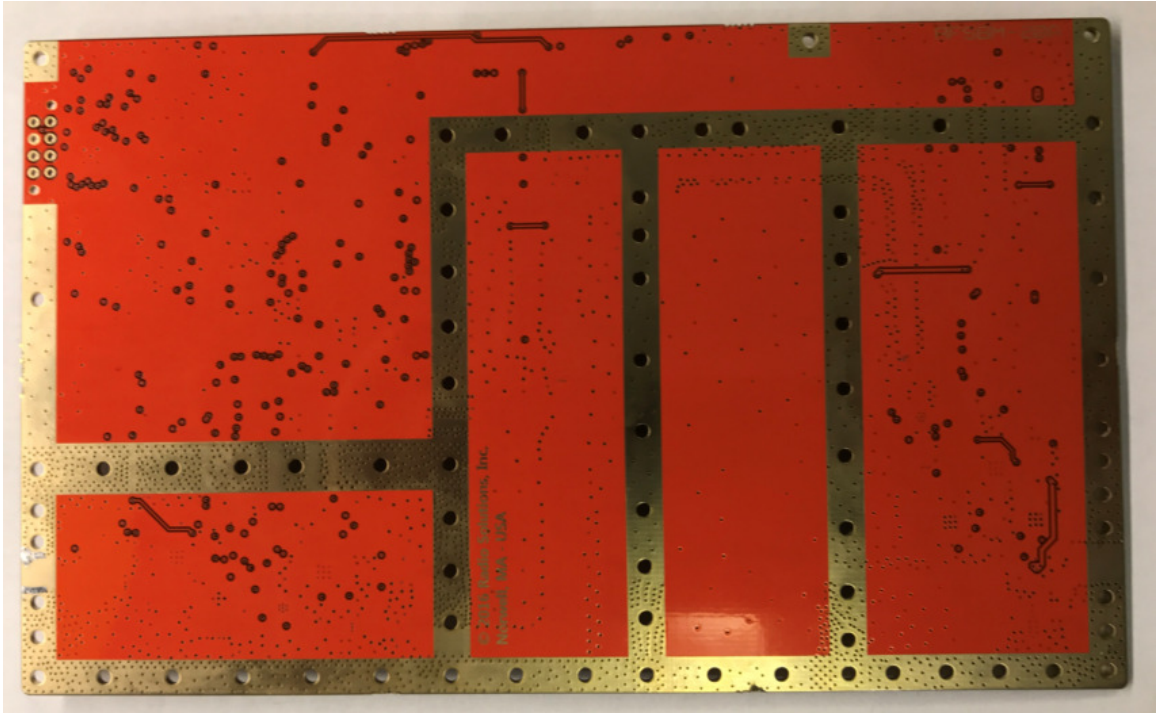
RF Module Back Side
