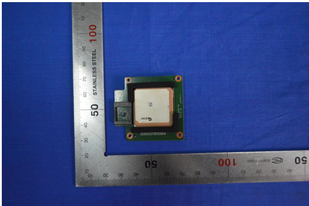
(4) EUT Photo
