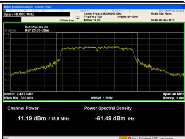
802.11g - AV Output power - CH11 2462
