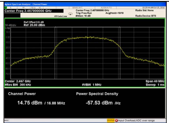
802.11b - AV Output power - CH12 2467
