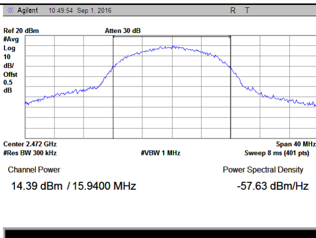
802.11b - AV Output power - CH13 2472
