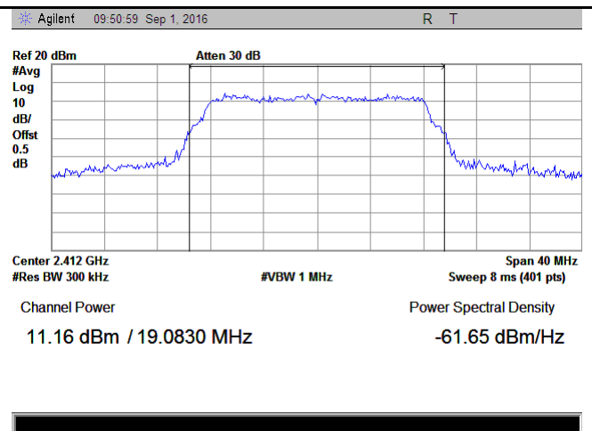
802.11g - AV Output power – CH1 2412
