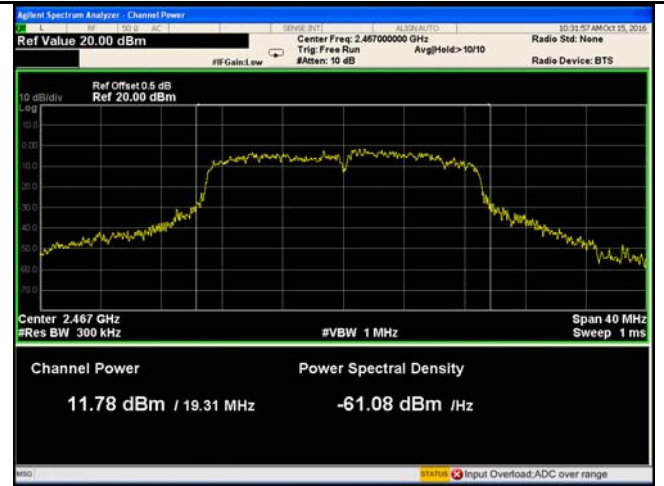
802.11n20 - AV Output power - CH12 2467
