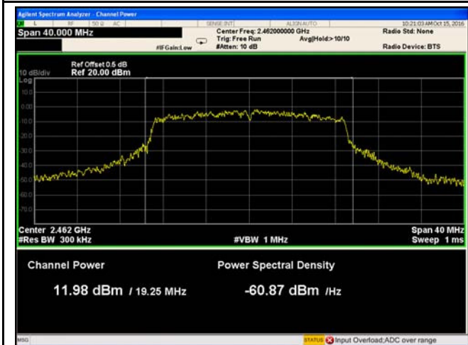
802.11n20 - AV Output power - CH11 2462
