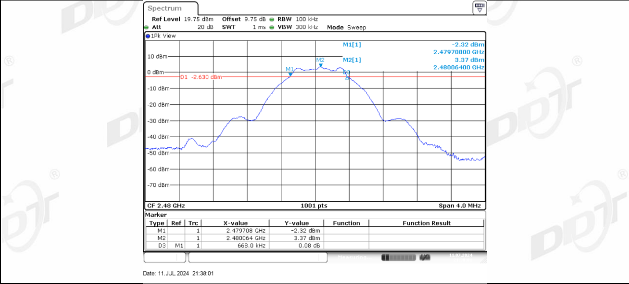
BLE_1M_Right side_2480
