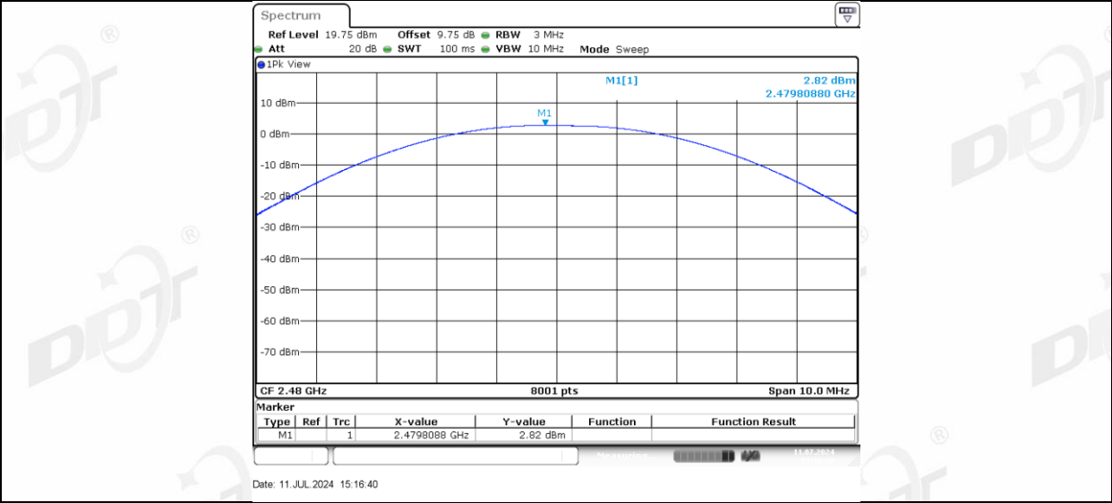
BLE_1M_Right side_2480
