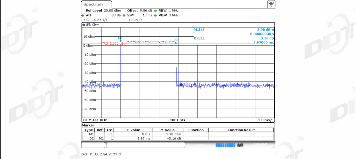
2DH5_Right side_Hop
