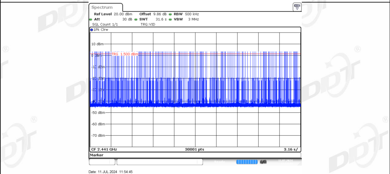
DH3_Right side_Hop
