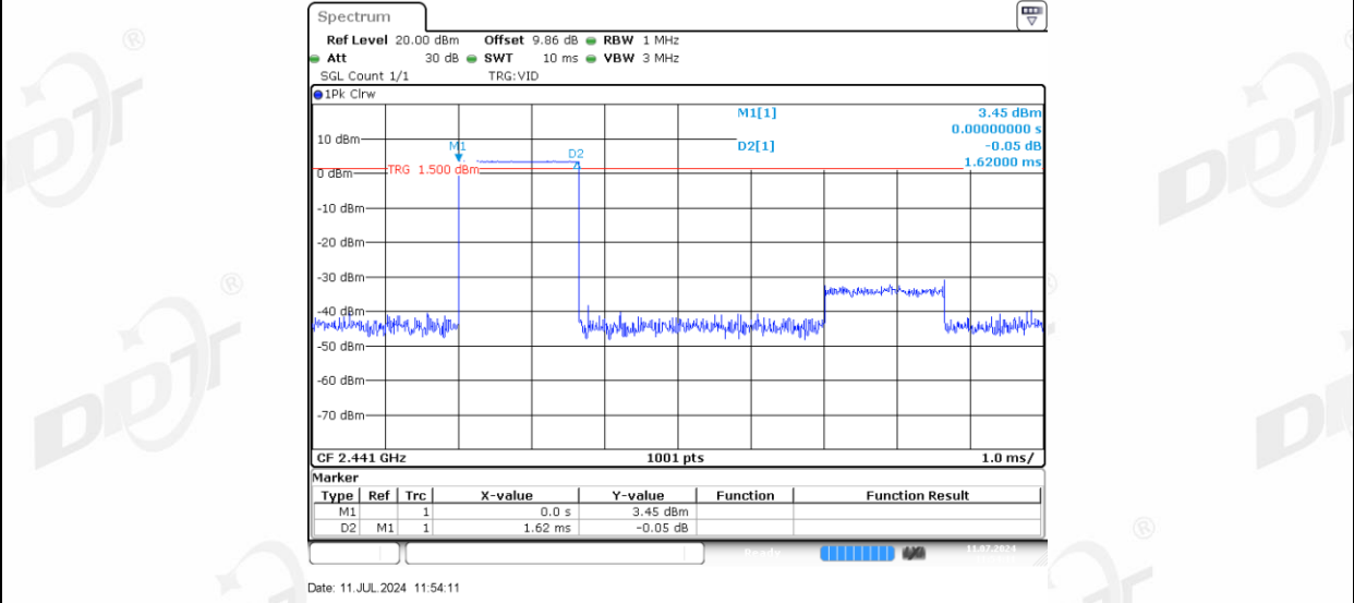
DH3_Left side_Hop
