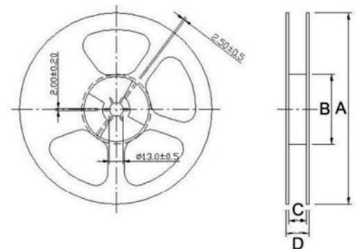
Reel Dimensions
