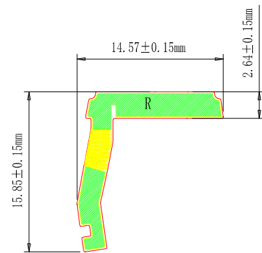
R 边天线尺寸图
