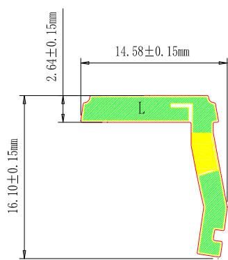
L 边天线尺寸图
