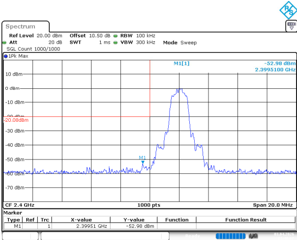
2EDR_2DH1_Low
