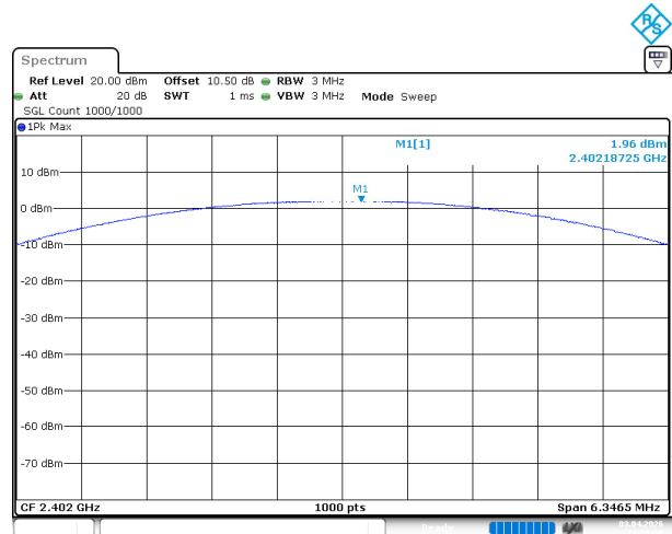
2EDR_2DH1_Low
